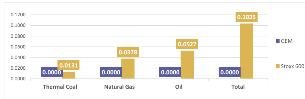
Emissions potentielles provenant de réserves d'énergies fossiles (MtCO 2 )
